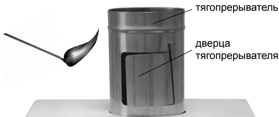
Рисунок 7. Тягопрерыватель
